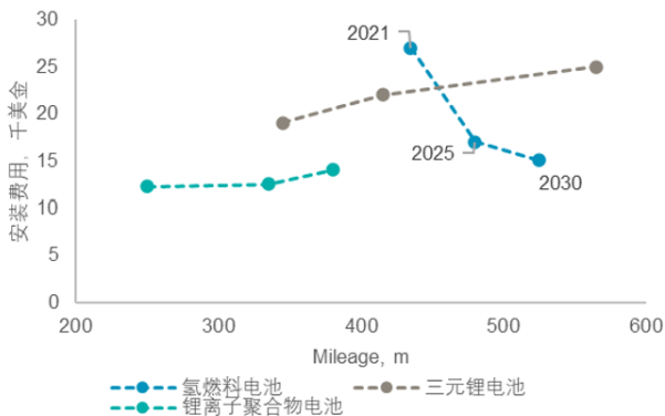
图 3: 氢燃料电池汽车的每英里成本经济受益于续航要求的增加，预示在高端 SUV 和轻型商用车市场有广泛的应用
