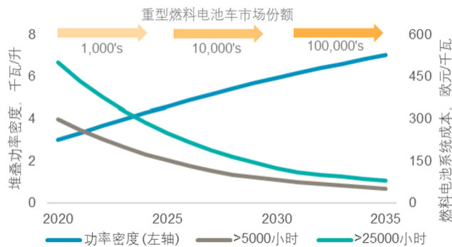
图 6: 提高功率密度有望降低燃料电池系统成本，推动市场应用
